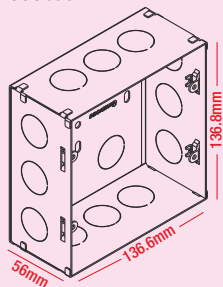
8 module (Vertical) 800177
