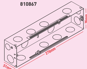
9 module 810867
