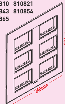
18 module 800180
