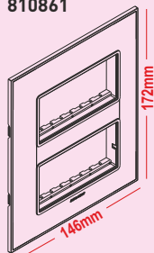
8 module (Vertical) 810806 810817 810839 810850 810861
