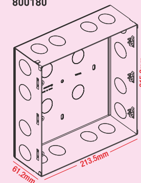
18 module 800180
