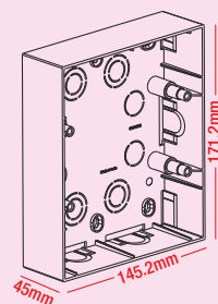
8 module (Vertical) 800187
