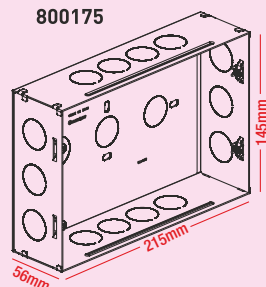
12 module 800175
