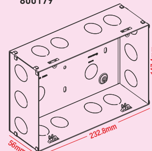
16 module 800179
