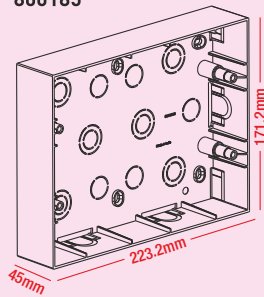
12 module 800185
